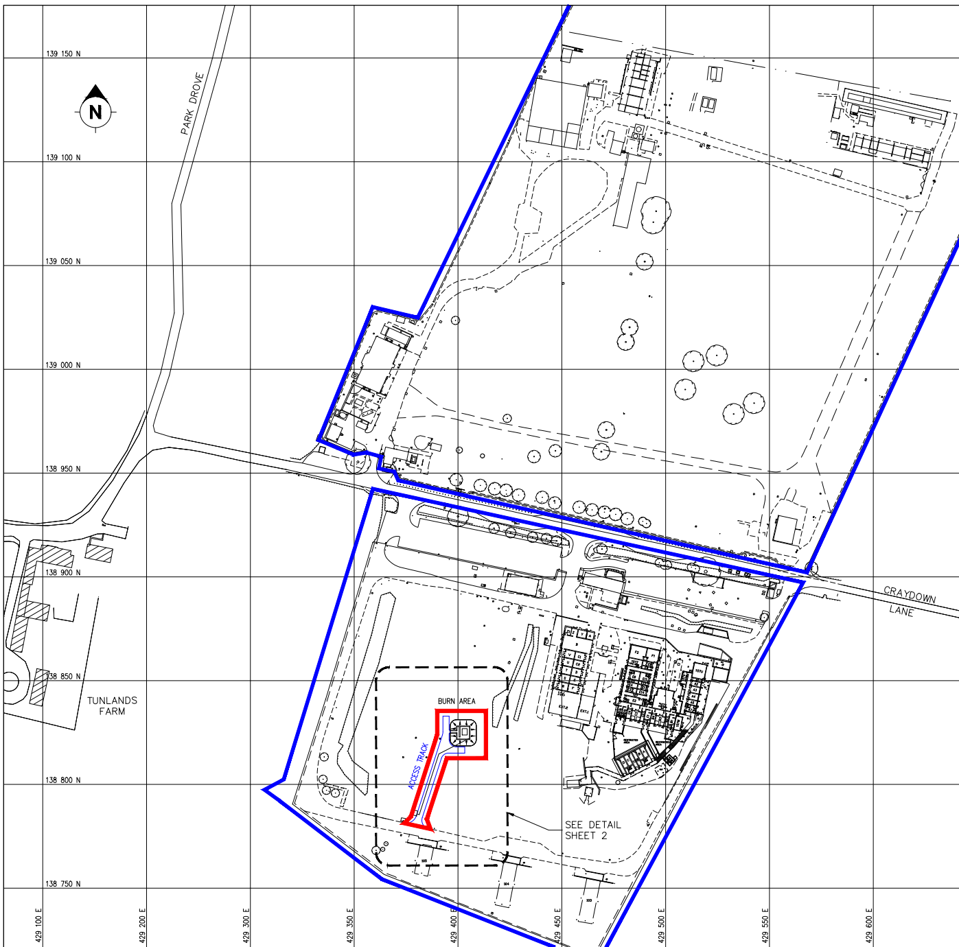
SITE PLAN (1:2500)
